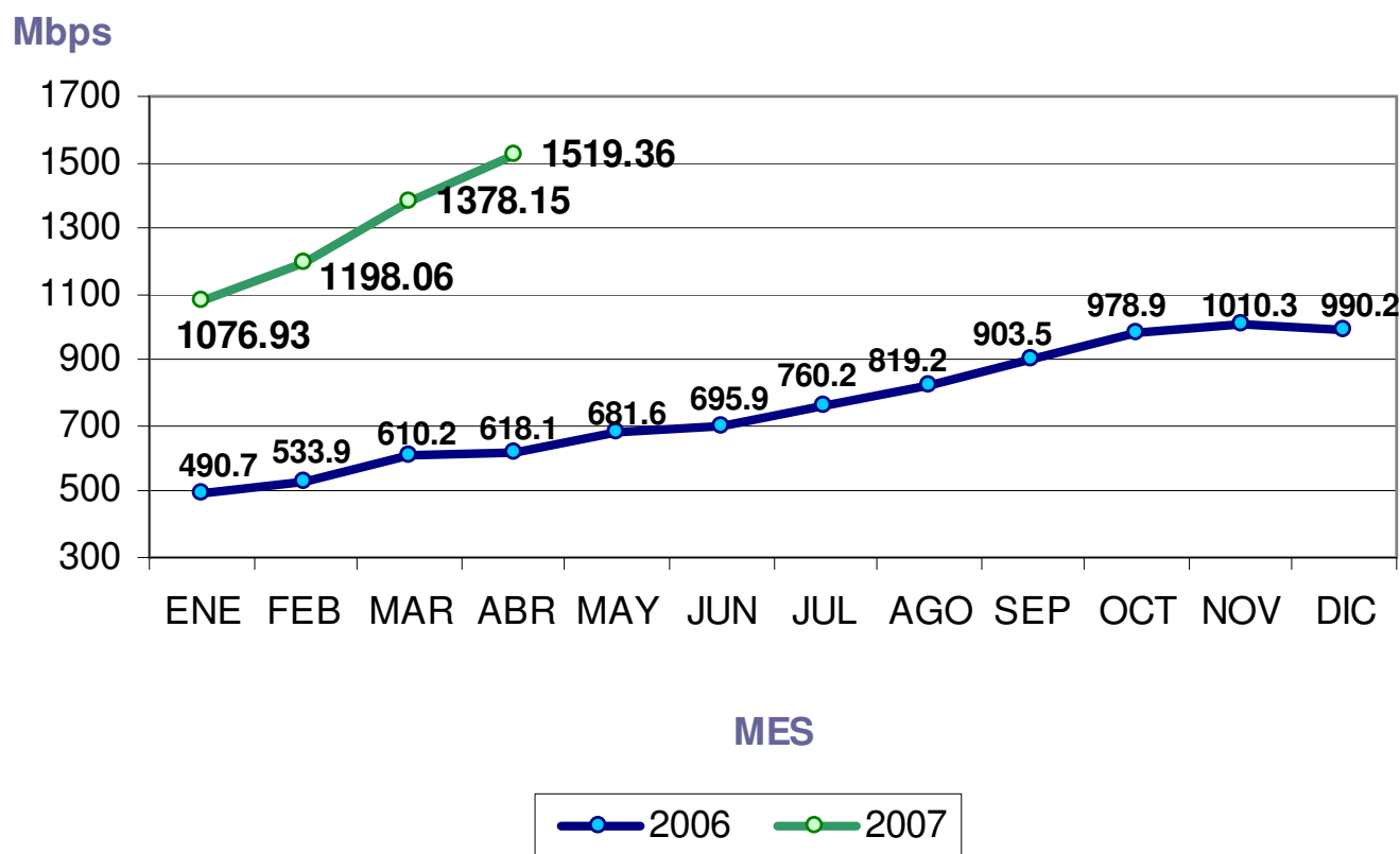
MAXIMOS VALORES MENSUALES DE TRAFICO DOS ÚLTIMOS AÑOS
